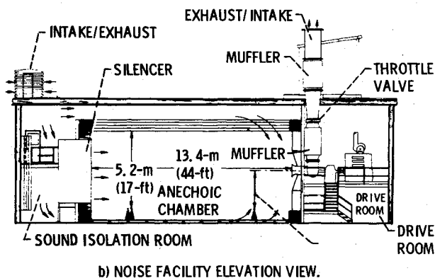
Fig. 2 Anechoic chamber.
