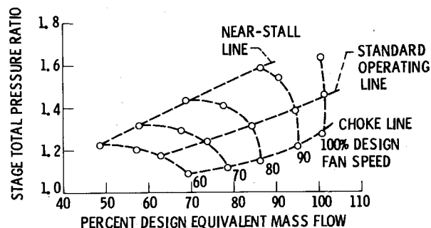
Fig. 7 Fan operating map.
